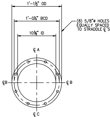
FLG DETAIL- ITEM #3
